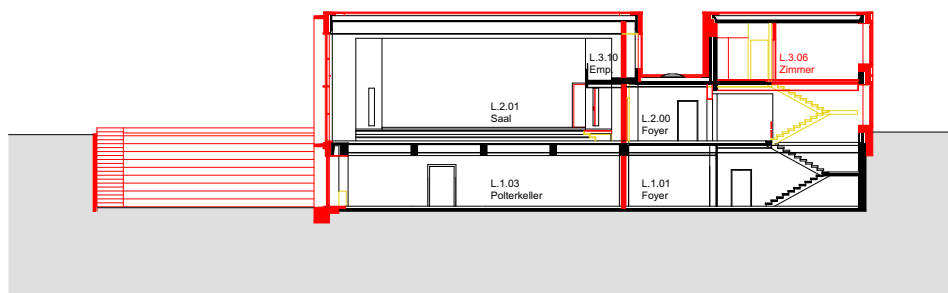
Schnitt L1
