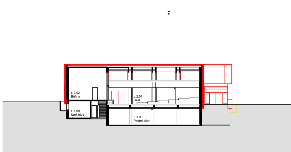
Schnitt L4
